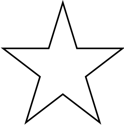
star
